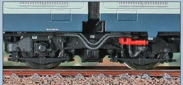
Dettaglio della riproduzione dei motori sui carrelli
